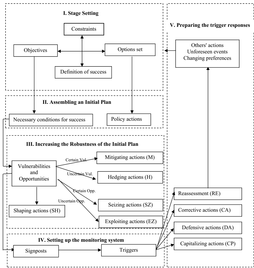
Fig. 3.1 Steps for DAP (Walker et al. 2013, p. 344)
